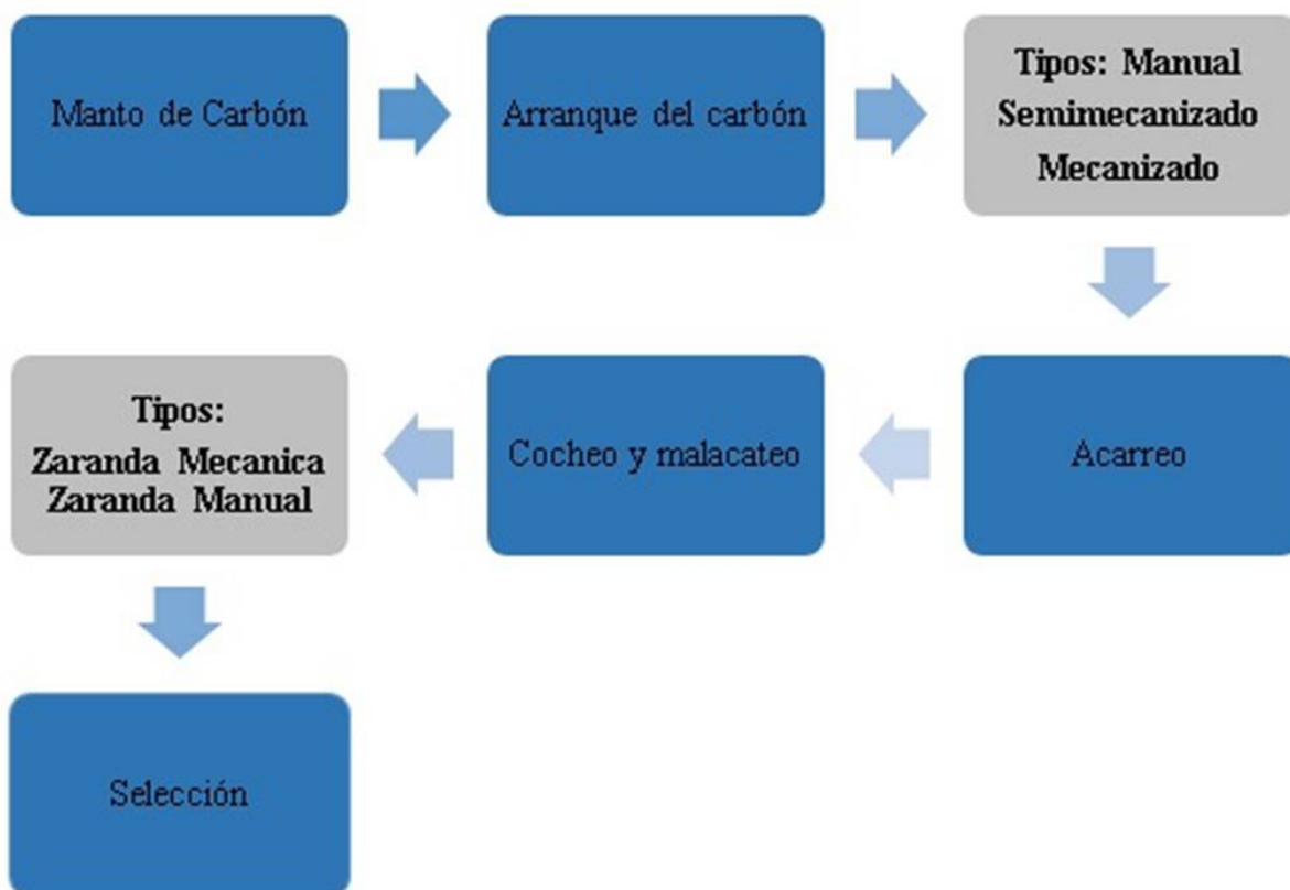
Figura 1 Procesos principales de producción de carbón a evaluar Fuente: los autores
