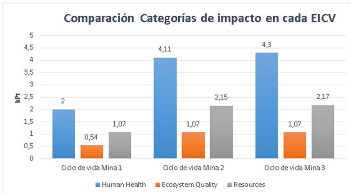
Figura 2 comparación categorías de impacto en los ciclos de vida de las tres minas Fuente: los autores
