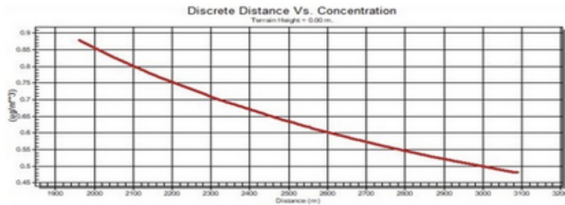
Figura 6 Dispersión de PM 10 desde las Caleras
