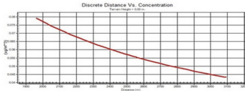
Figura 7 Dispersión de Cd desde las Caleras Fuente: los autores.
