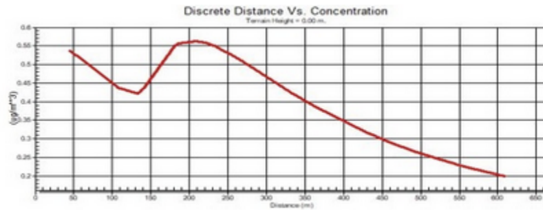
Figura 5 Dispersión de Cd desde la estación de bomberos Fuente: los autores.
