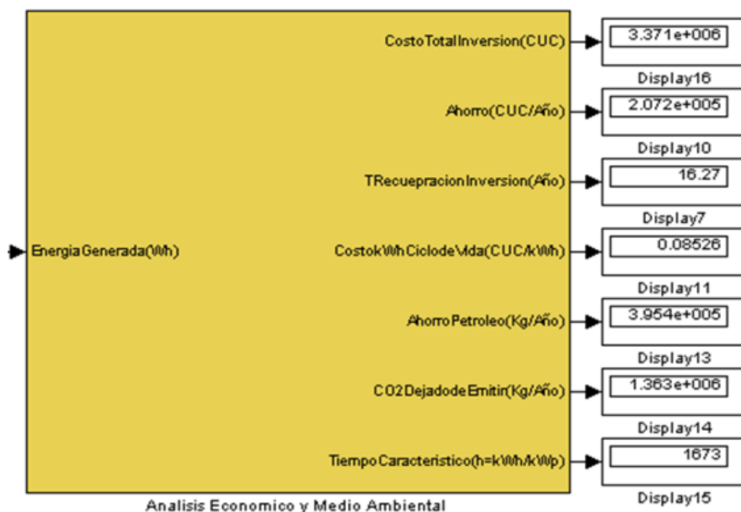
Fig.4. Resultados de la simulación del sistema para el bloque de análisis económico y medio ambiental.
