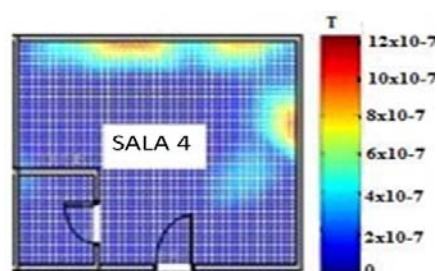
Fig.8. Representación de los valores promedios obtenidos en T en las mediciones en la sala 4 durante cinco días de medición.
