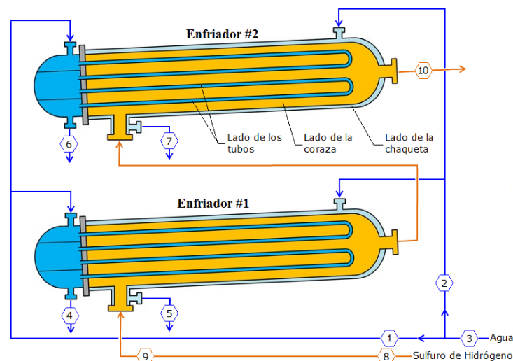
Fig. 1. Esquema de una pareja de enfriadores de sulfuro de hidrógeno y puntos de medición
