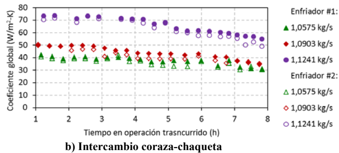
Fig. 2. Comportamiento del coeficiente global de transferencia de calor (método DTML)
