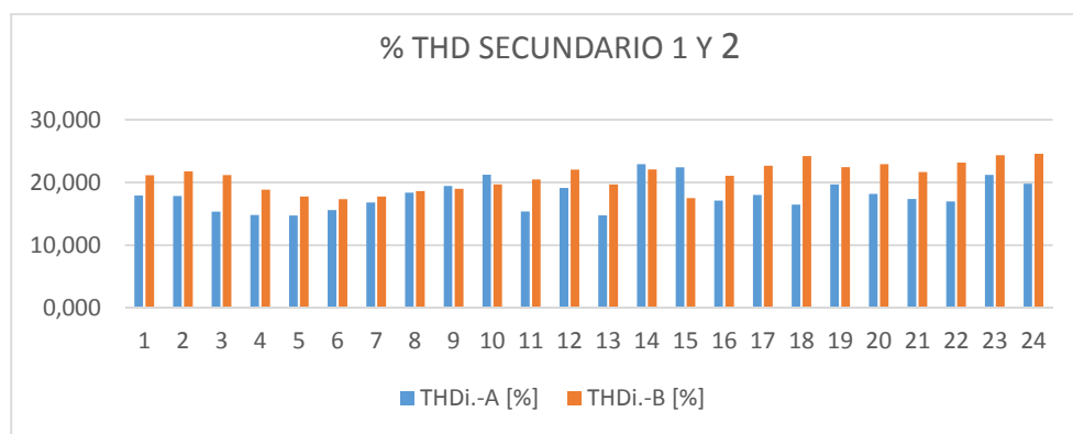
Fig. 1. THDI del transformador monofásico de 25kVA.
