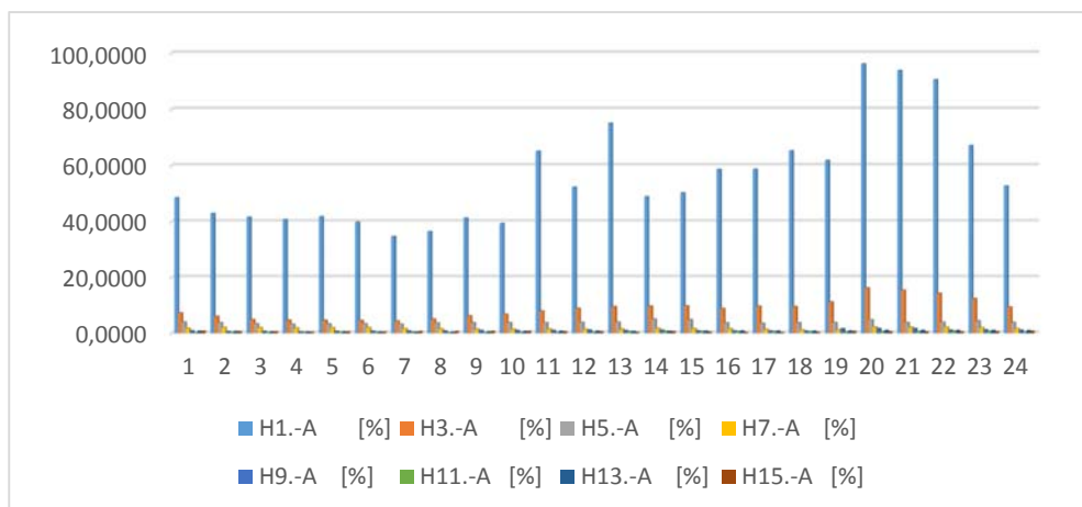
Fig. 2. Espectro armónico secundario 1.
