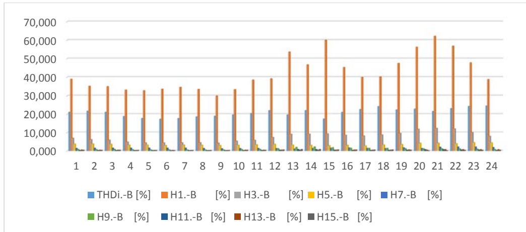
Fig. 3. Espectro armónico secundario 2.
