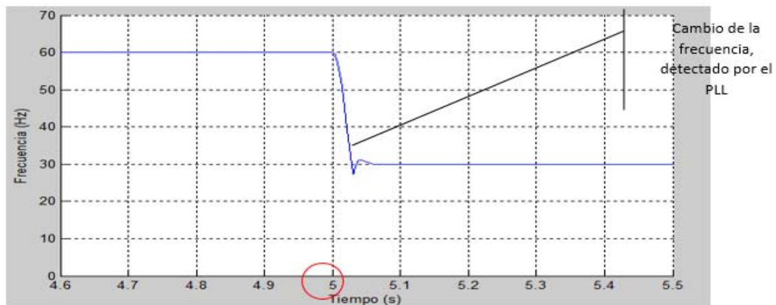
Fig. 2. Frecuencia muestreada por el PLL.
