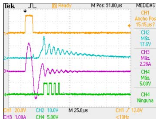
Fig. 10. Pulso de activación del IGBT inferior (amarillo), tensión rectificada de salida del condensador de desacople (azul), corriente en la carga (rosado) y tensión de salida del comparador analógico, con recipiente de aluminio con fondo ferromagnético empotrado.
