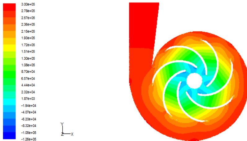
Fig. 8. Distribución de presión en la bomba.
