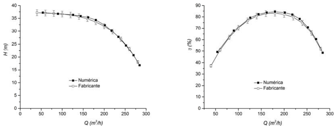
Fig. 5. Comparación de los resultados numéricos vs experimentales del fabricante; a) Carga versus flujo, b) Eficiencia versus flujo.
