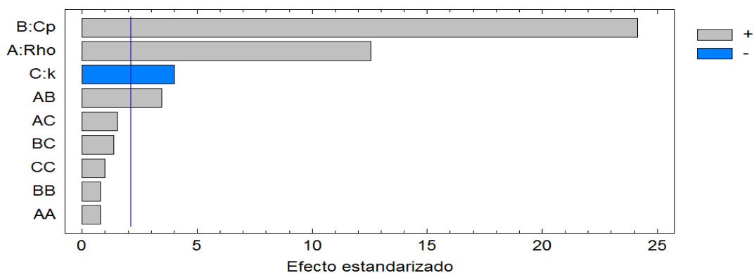
Fig. 1. Carta de Pareto estandarizada para el tiempo de enfriamiento.
