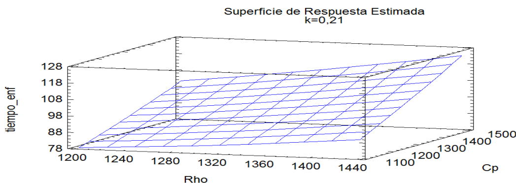
Fig. 2. Superficie de respuesta estimada.
