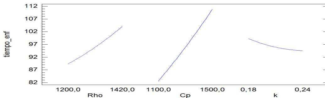
Fig. 3. Gráfica de Efectos Principales para tiempo de enfriamiento.
