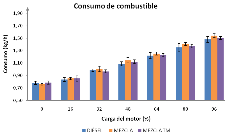
Fig. 7 Comportamiento del consumo horario de combustible.
