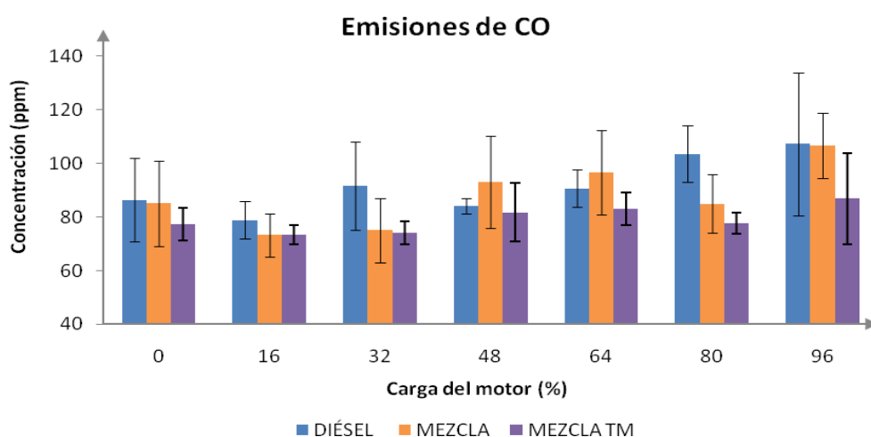
Fig. 4 Comportamiento de las emisiones de CO.
