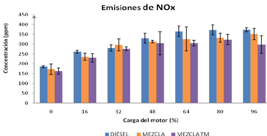
Fig. 6 Comportamiento de las emisiones de NOx.
