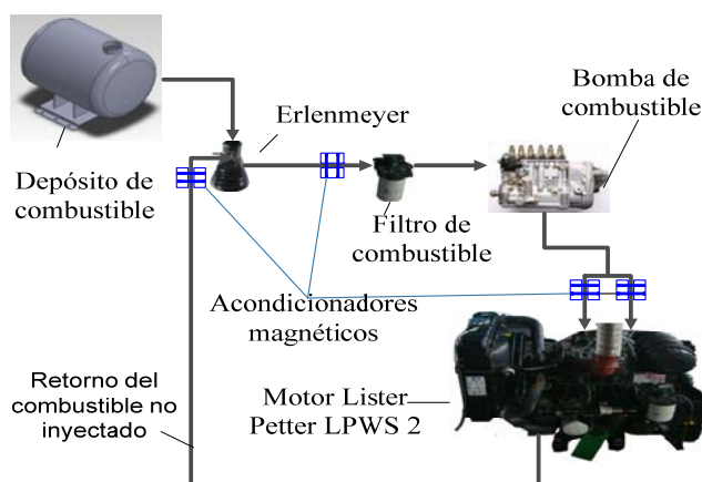
Fig. 2 Diagrama descriptivo con la ubicación de los acondicionadores magnéticos en el motor.
