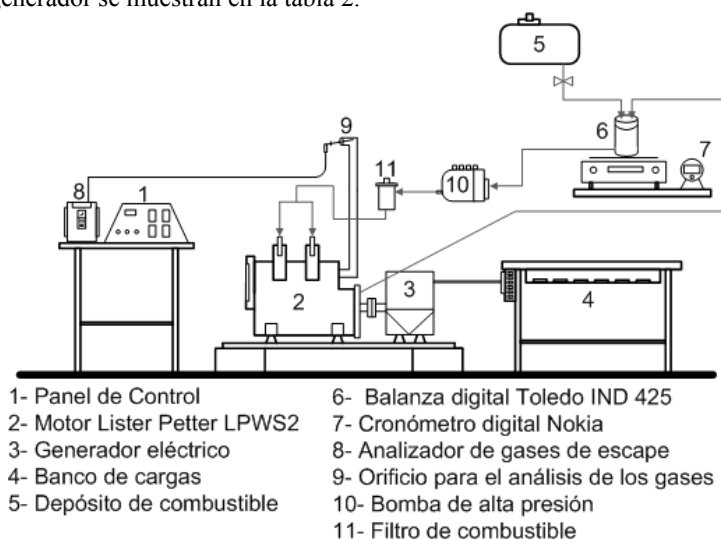
Fig. 1. Diagrama esquemático de la instalación experimental.
