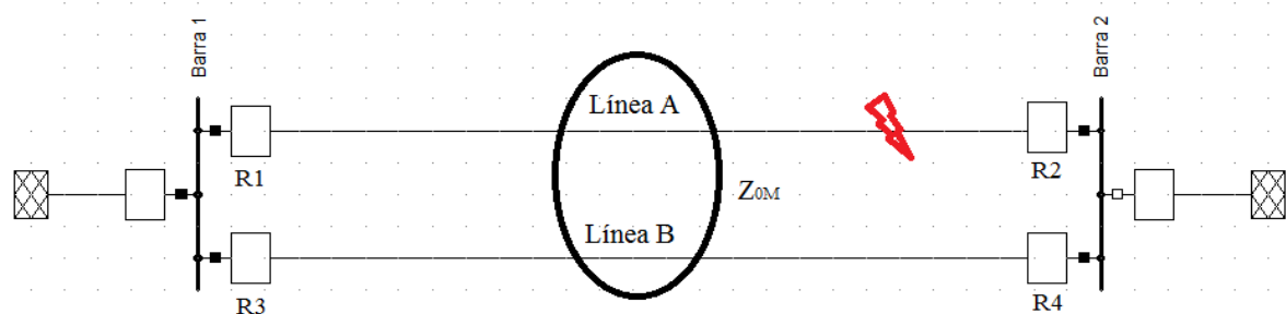
Fig. 3. Sistema a 110 kV en ambiente de DigSilent Power Factory, con acoplamiento mutuo entre las líneas paralelas A y B, con relés 21N y 67N en R1, R2, R3 y R4.
