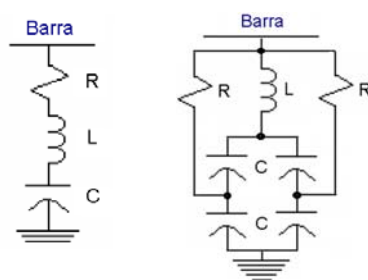
Fig. 5. Esquemas simplificados de los diferentes filtros de armónicos [1].
