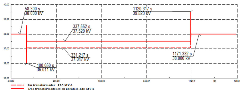
Fig. 8. Comportamiento de la tensión secuencia positiva sin instalar los filtros, ni SVC, ni BESS.
