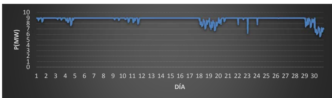
Fig. 6. Potencia activa entregada al SEN. Fuente: Elaboración Propia.
