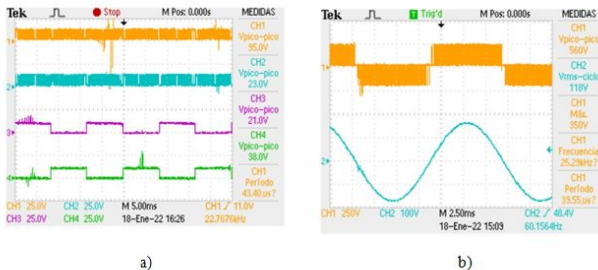
Fig. 8.a) Señales de control de los transistores b) Tensión de salida delinversor
