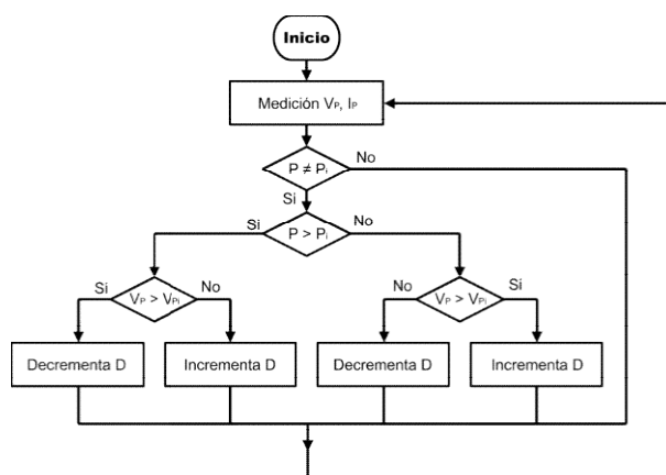
Fig. 5. Diagrama en Bloques del Algoritmo MPPT
