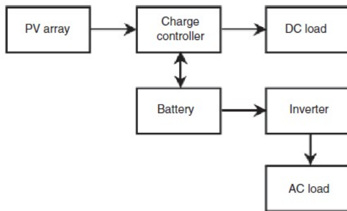
Fig. 1. Diagrama en bloques de un sistema fotovoltaico autónomo [7]
