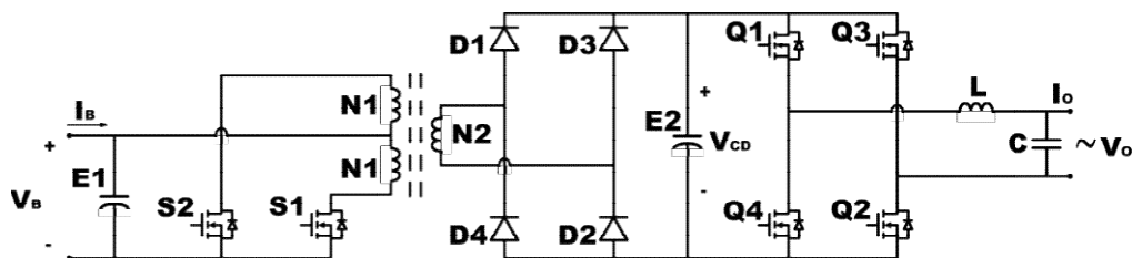
Fig. 4. Convertidores de la etapa inversora
