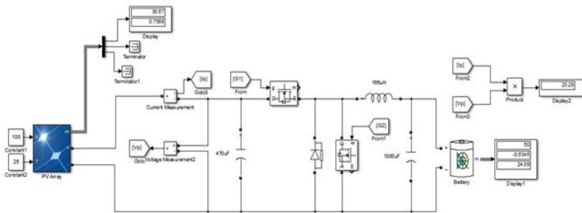
Fig. 9. Modelo y simulación en MATLAB del regulador de carga para una Irradiancia de 1000W/m 2
