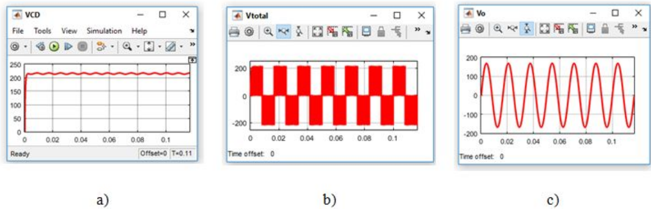
Fig. 13 a) Tensión a la salida del convertidor Push-Pull b) Tensión en el inversor sin filtrar c) Tensión de salida del sistema
