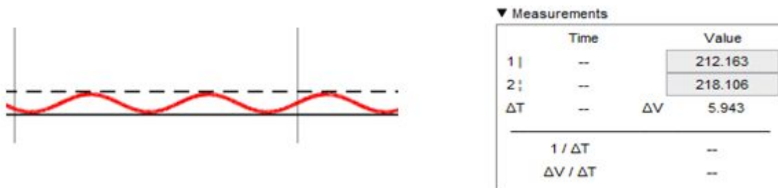
Fig. 14. Tensión de rizado a la salida del Push-Pull
