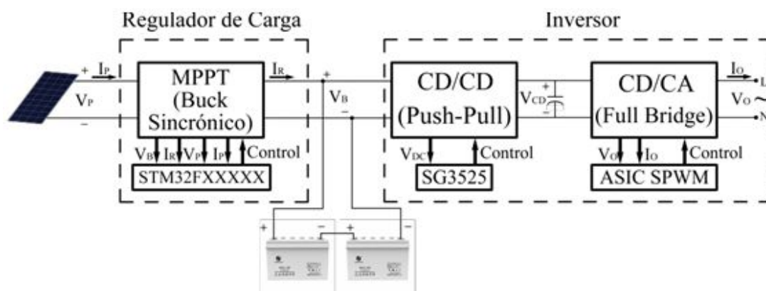
Fig. 2. Convertidores Electrónicos de Potencia utilizados
