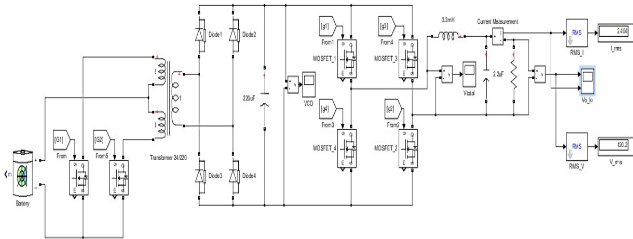
Fig. 12. Modelo en MATLAB de la etapa inversora
