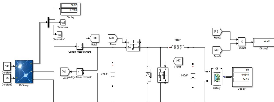
Fig. 10. Modelo y simulación en MATLAB del regulador de carga para una Irradiancia de 100W/m 2
