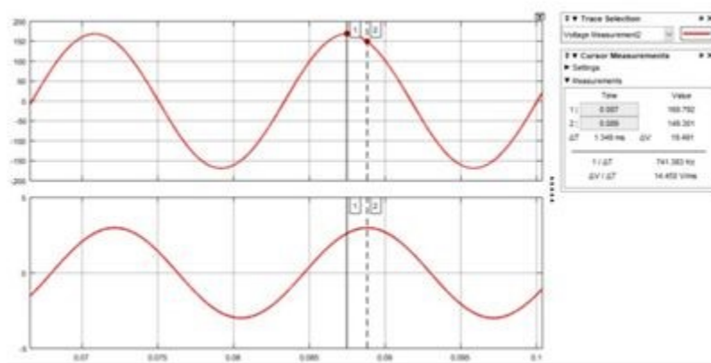
Fig. 15. Tensión y corriente a la salida con carga R-L
