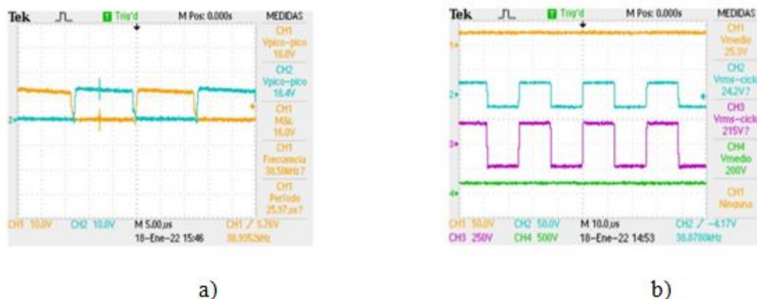
Fig. 7. a) Señales de control de los transistores S1 y S2 b) Tensión a la entrada, Tensión en elprimarioy secundario del transformador y a la salida del Push-Pull
