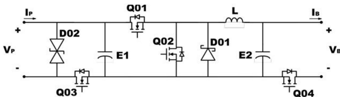
Fig. 3. Esquema del convertidor Buck Sincrónico
