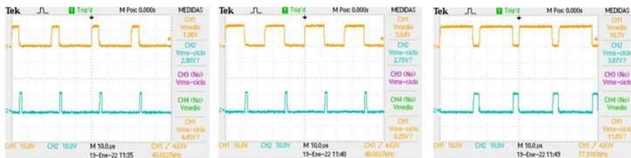
Fig. 6. Señales de control de Q01 y Q02 durante el proceso de búsqueda del punto de máxima potencia
