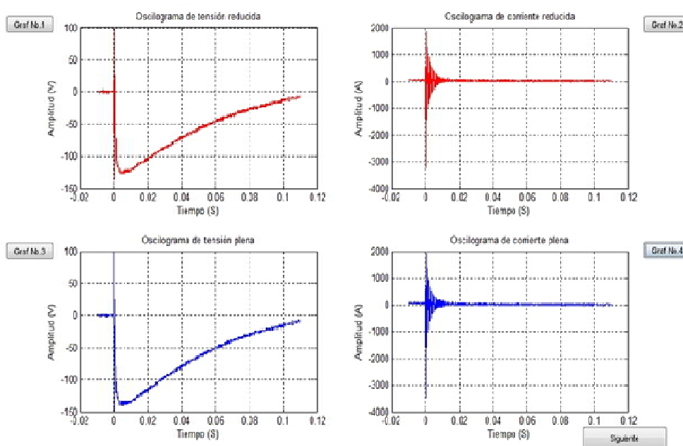
Fig. 8. Oscilogramas en el dominio del tiempo por terminal H_1
