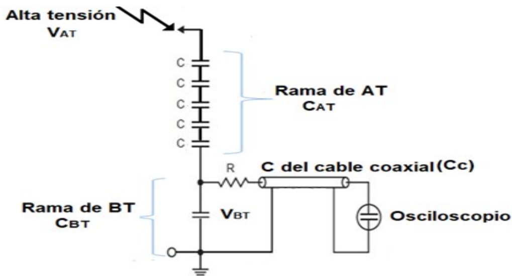
Fig. 3. Divisor capacitivo del generador de impulsos
