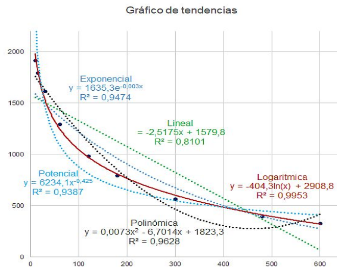
Fig. 3. Líneas de tendencia, ecuaciones características y valor de varianza explicado por el modelo (R2) para el modelo A602/3300
