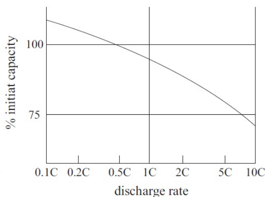
Fig. 2. Efecto de la corriente de descarga en la capacidad de descarga [9]
