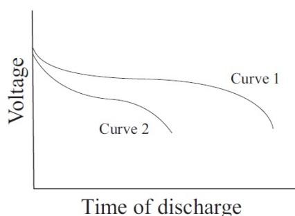
Fig. 1. Efecto de la corriente de descarga en la caída del voltaje [9]
