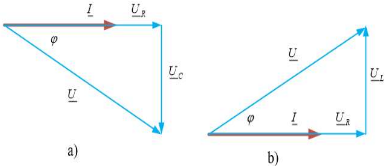
Fig. 3. Representación de los diagramas fasoriales a) circuito RC, b) circuito RL. (Fuente: elaboración propia)
