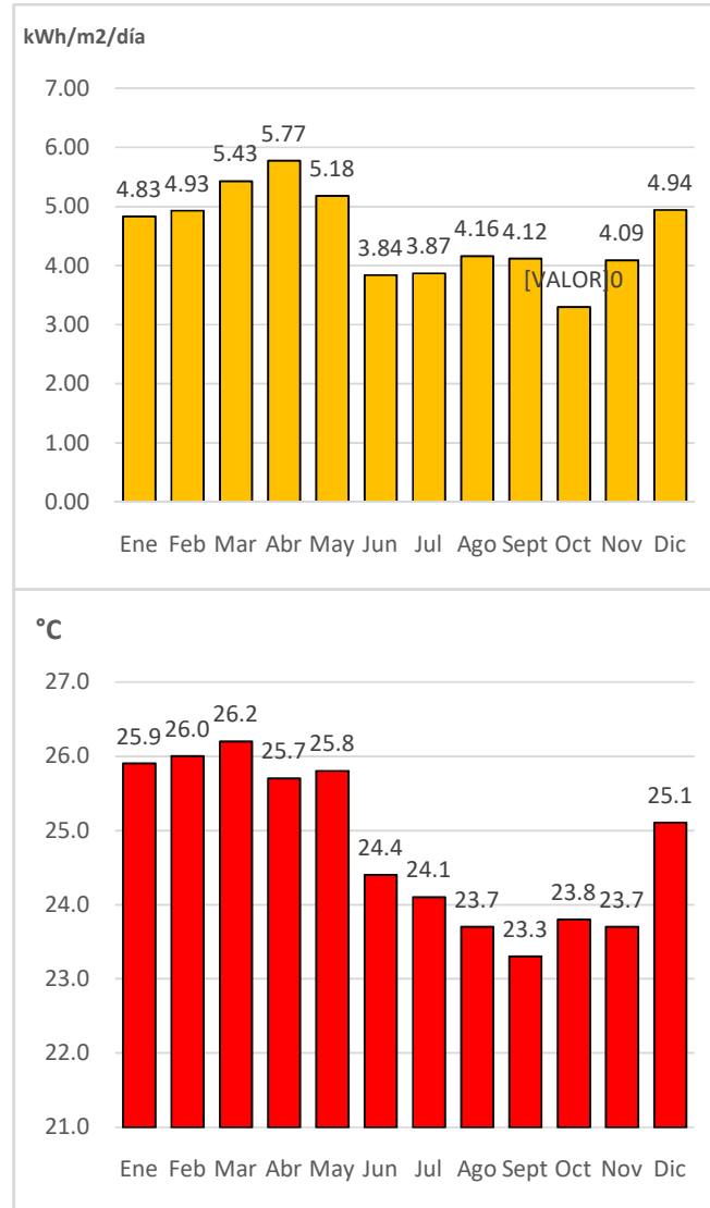
Fig. 3. IGH y temperatura ambiente en la zona de estudio determinadas con la base de datos Meteonorm 8,0
