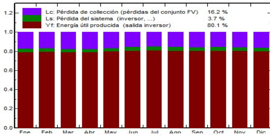
Fig. 5. Producción normalizada y factores de pérdida
