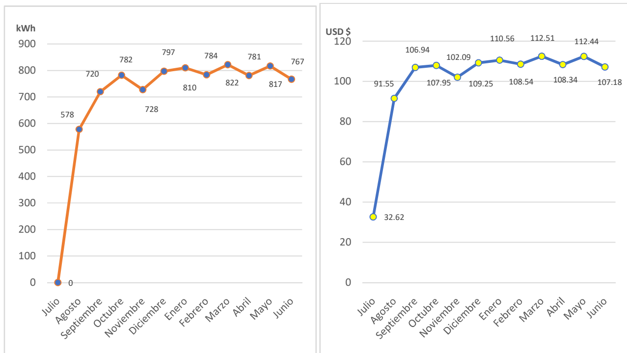
Fig. 2. Perfil de carga y pago por consumo 2021-2022, respectivamente
