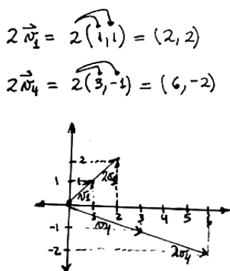
Figura 7. E3 generando la construcción de vectores que se estiran y contraen, como una función.
