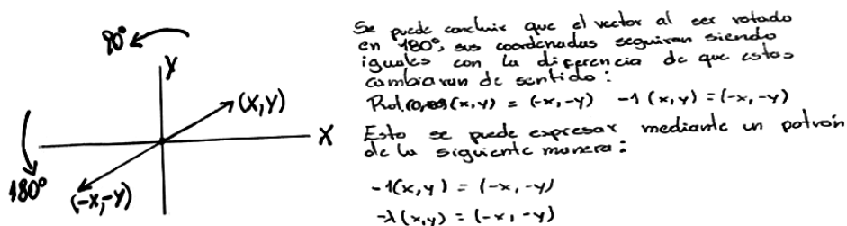
Figura 6. E3 determinando vectores a través de una Rotación en 180^\circ
