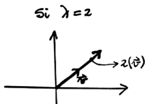
Figura 4. E2 interpretando el múltiplo escalar de un vector v
