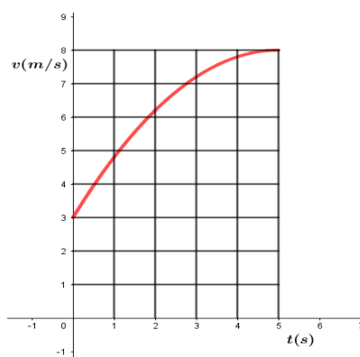
Figura 4. Estimación de la distancia recorrida por un móvil. (Elaboración propia. Inspirado en Stewart, 2012a, p. 369)
