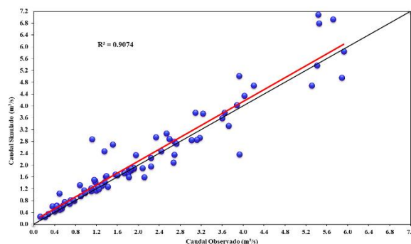
Figura 4. Correlación lineal entre el caudal simulado con el modelo PRMS IV con respecto al caudal observado medidos en la bocatoma Apacheta.
