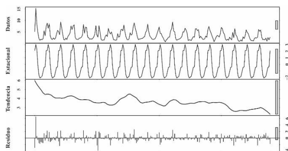
Figura 9. Descomposición de la serie de tiempo del caudal medio mensual de salida simulado con PRMS-IV en la microcuenca Apacheta, desde el año 2000 al 2018.
