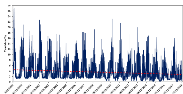
Figura 5. Serie de tiempo del caudal diario de salida simulado con el modelo PRMS-IV en la microcuenca Apacheta, del año 2000 al 2018.
