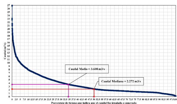
Figura 6. Curva de Duración de Flujo para el caudal de salida simulado con PRMS-IV en la bocatoma Apacheta, del año 2000 al 2018.
