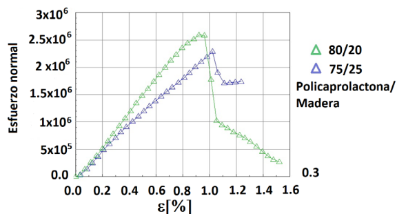
Figura 4. Curvas esfuerzo-deformación de la prueba de flexión a tres puntos para las muestras.
