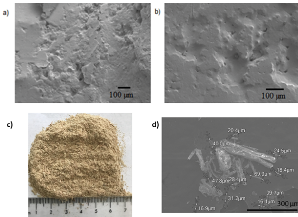
Figura 1. Micrografías de SEM de a) 75/25, b) 80/20 policaprolactona/harina de álamo, c) fotografía de harina de álamo y d) micrografía de la harina de álamo.
