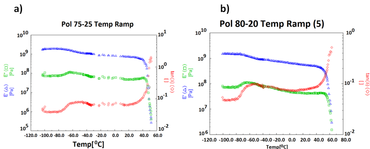
Figura 5. Barrido de temperatura para las muestras a) 75/25 y b) 80/20 Policaprolactona/harina de álamo.
