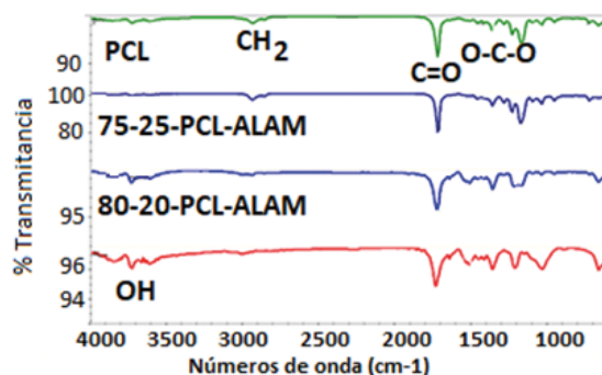
Figura 2. Espectros de infrarrojo de los materiales compuestos.
