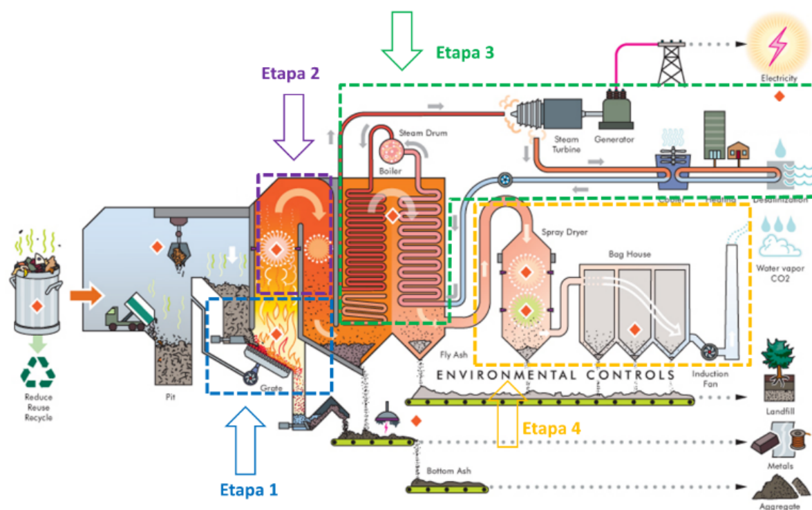
Figura 1. Esquema del proceso de incineración de RSM en parrilla (adaptado de [9]). Etapa 1: combustión de RSM, etapa 2: post-combustión y reducción de NO x , etapa 3: generación de vapor y potencia, etapa 4: control ambiental.
