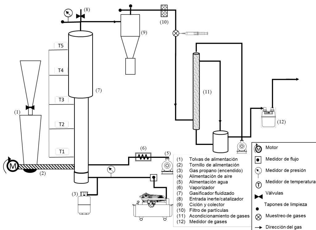
Figura 1. Esquema del sistema de gasificación a escala banco.
