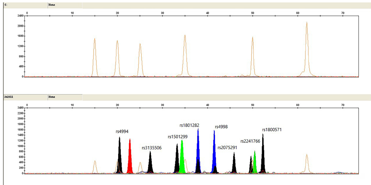
Figura 3: Arriba: Electroferograma de un control negativo con el marcador de peso molecular GeneScan™ 120 LIZ™. Abajo: Electroferograma de un control positivo donde se visualiza el perfil genético de los polimorfismos de los genes ADBR3 ( rs4994 ; rs4998 ), APOA5 ( rs3135506 ; rs2075291 ), ADIPOQ ( rs1501299 , rs2241766 ) y PPARG ( rs1801282 , rs1800571 ).
