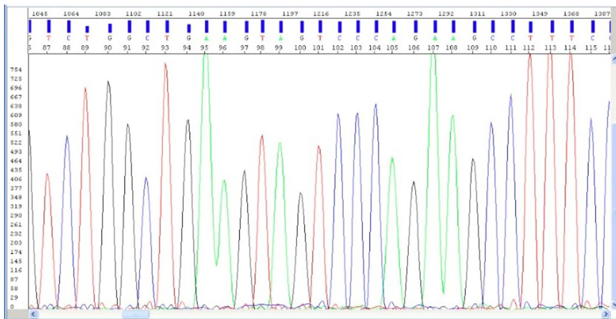
Figura 1. Resultado de la secuenciación directa de un segmento del gen APOA.
