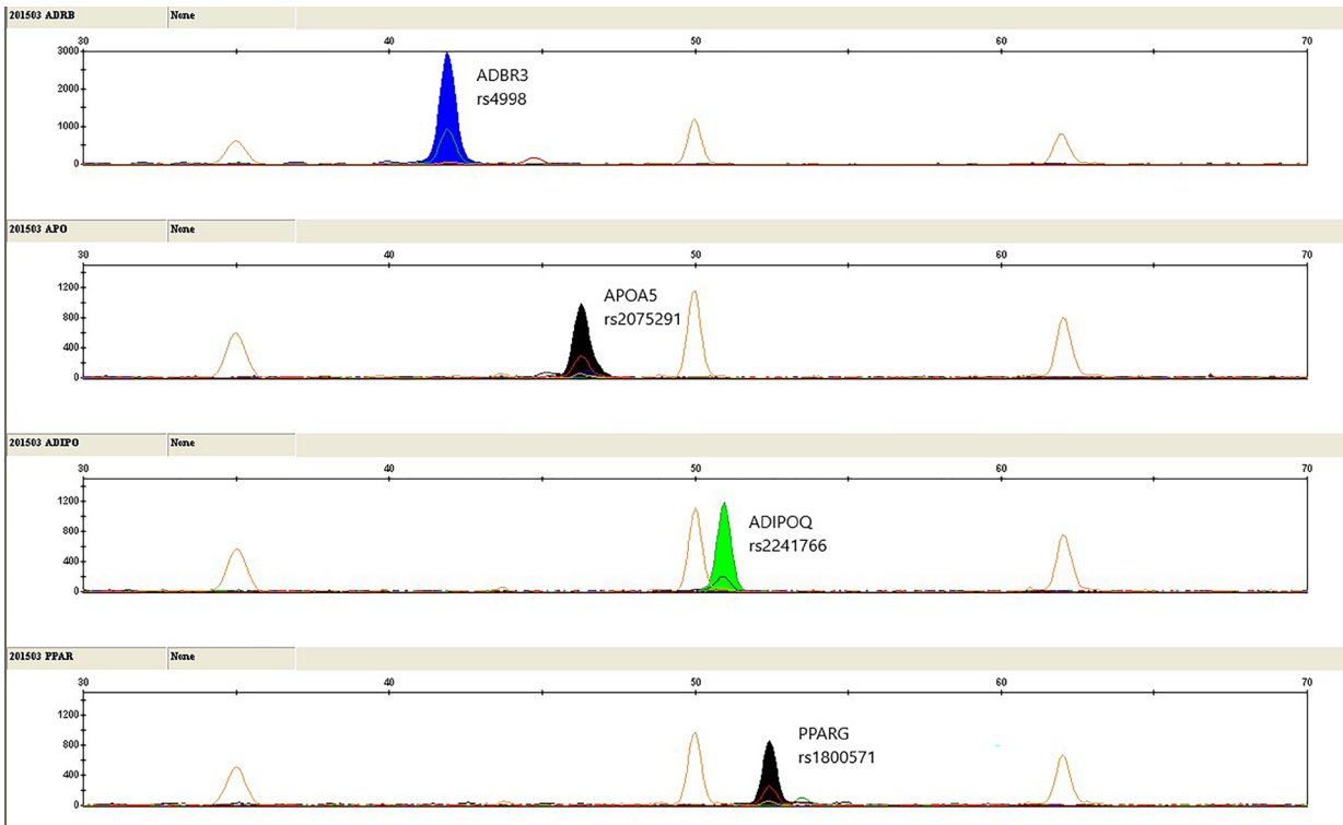
Figura 2. Identificación de cuatro polimorfismos amplificados en forma individual.
