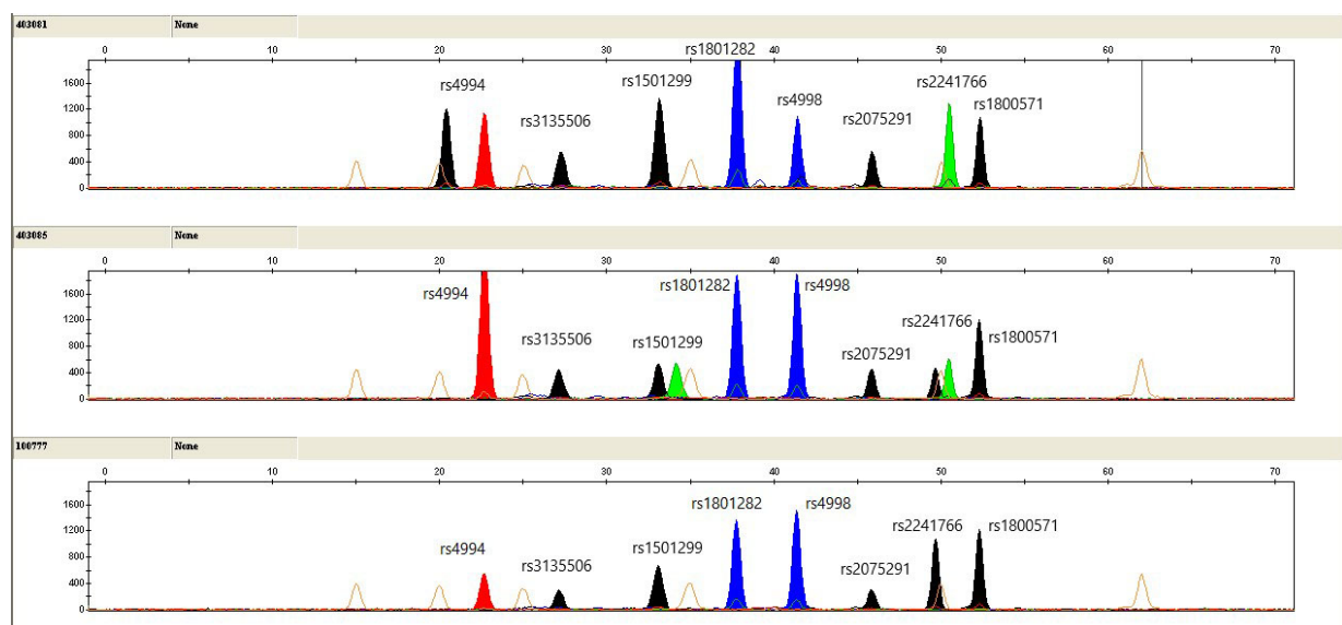
Figura 4. Electroferogramas obtenidos de tres muestras analizadas. Se visualiza el perfil genético de los polimorfismos de los genes ADBR3 ( rs4994 ; rs4998 ), APOA5 ( rs3135506 ; rs2075291 ), ADIPOQ ( rs1501299 , rs2241766 ) y PPARG ( rs1801282 ; rs1800571 ).
