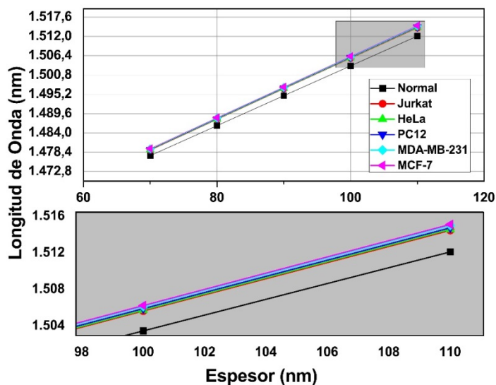
FIG. 5. Variación de los picos de resonancia en función del espesor de la nano cavidad TE con ángulo de incidencia 75^\circ Fuente: elaboración propia.
