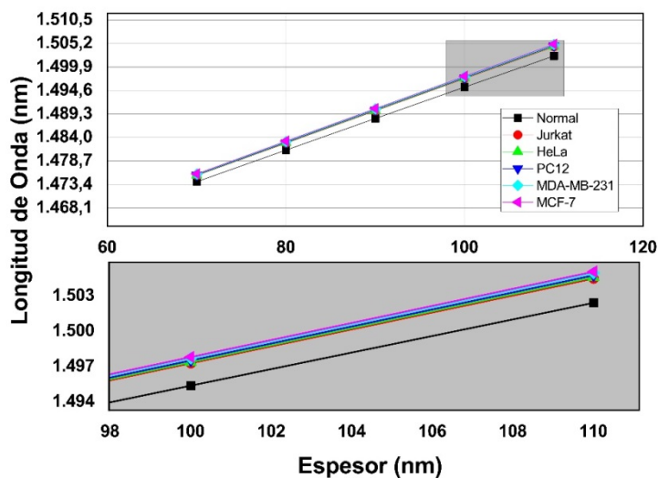
FIG. 6. Variación de los picos de resonancia en función del espesor de la nano cavidad TM con ángulo de incidencia 50^\circ Fuente: elaboración propia.
