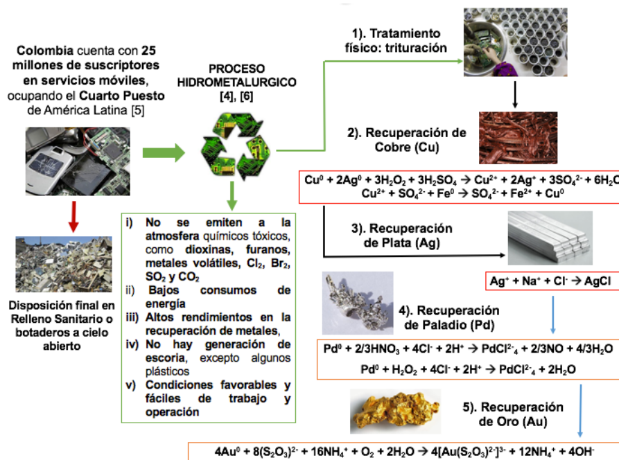
FIGURA 4. Metodología para la recuperación de metales preciosos y de interés industrial a partir de WEEE y empleando un proceso hidrometalúrgico Fuente: elaboración propia.
