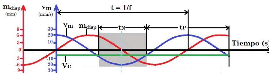
FIGURA 9. Vibraciones en el molde de colada continua.
