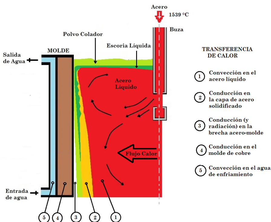
FIGURA 2. Transferencia de calor en el molde.
