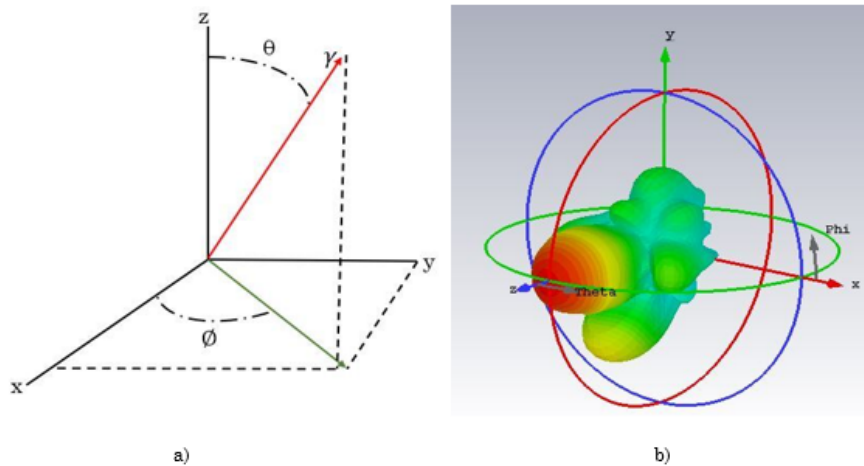
FIGURA 12. Diagramas de radiación de una antena, a) representación bidimensional y b) representación en un modelo 3D.
