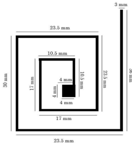
FIGURA 3. Dimensiones de ranura espiral en parche radiante. Fuente: elaboración propia.
