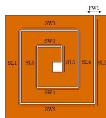
FIGURA 2. Dimensiones de ranura espiral en parche radiante.
