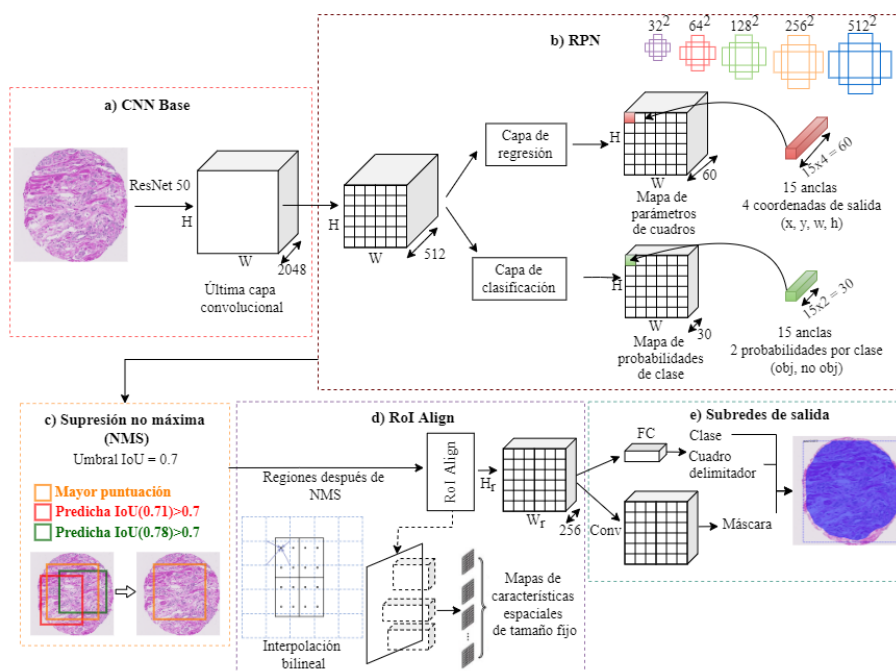
FIGURA 2. Método Mask R-CNN para la segmentación de instancias
