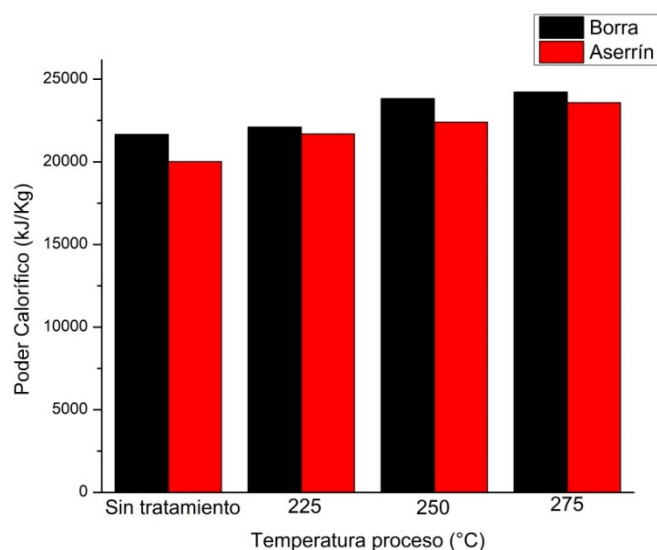
FIGURA 5. Poder calorífico de biomásas del aserrín y de la borra de café
