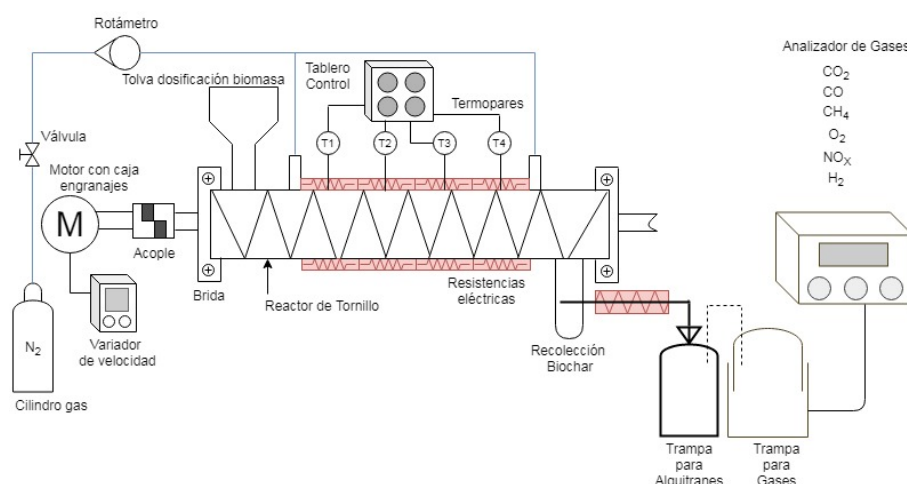
FIGURA 1. Esquema y fotografía del reactor de torrefacción de tornillo Fuente: elaboración propia.
