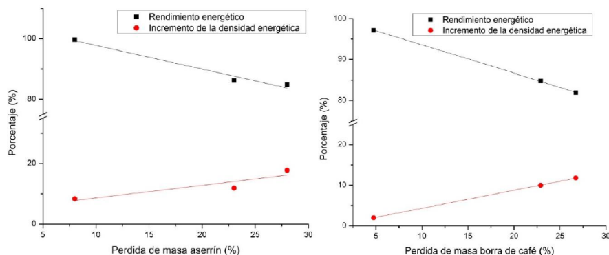
FIGURA 6. Variación del rendimiento energético y la densidad energética con la pérdida de masa durante la torrefacción del aserrín y borra de café
