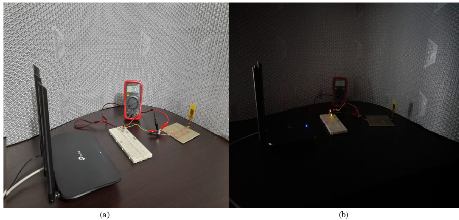
FIGURA 15. (a) Captación de energía RF con la rectenna propuesta logrando 3.02 V de carga. (b) Prueba del sensor de oscuridad
