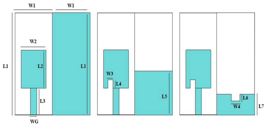
FIGURA 2. Proceso de diseño de la antena monopolo propuesta Fuente: Elaboración propia.
