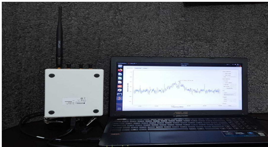
FIGURA 8. Toma de medidas de intensidad de señal con la antenna VERT2450 Fuente: Elaboración propia.
