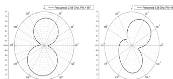
FIGURA 5. Patrones de radiación de la antena propuesta Fuente: Elaboración propia.
