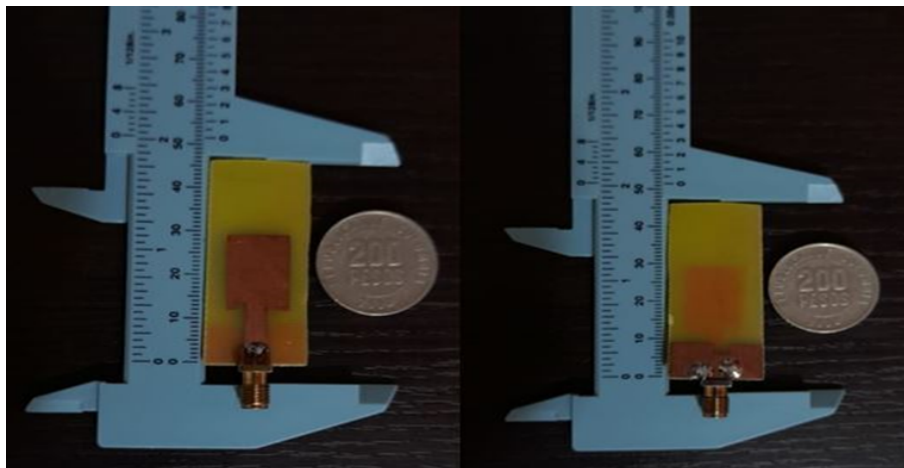
FIGURA 3. Antena fabricada Fuente: Elaboración propia.
