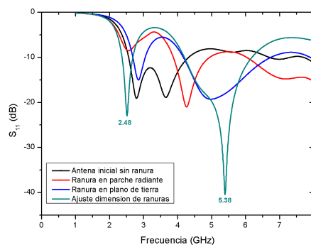
FIGURA 4. Coeficiente de reflexión ( S_{11} ) del proceso de evolución de la antena propuesta Fuente: Elaboración propia.
