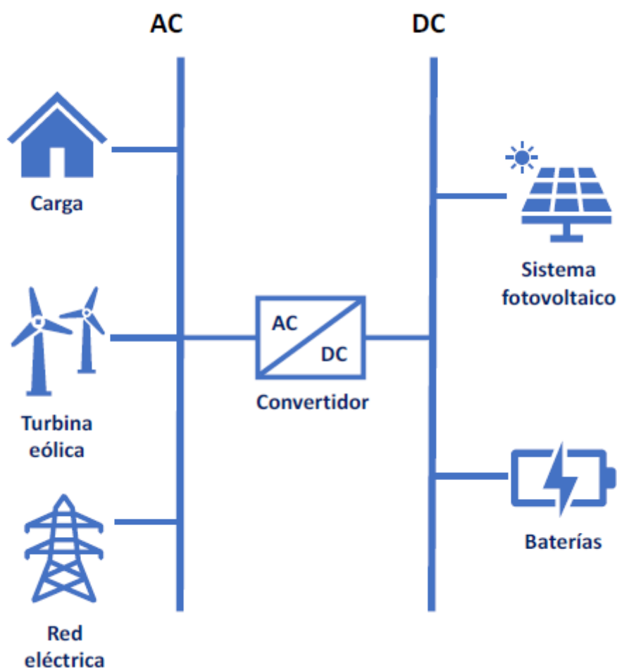
Figura 1 Esquema de microrred Fuente: elaboración propia.
