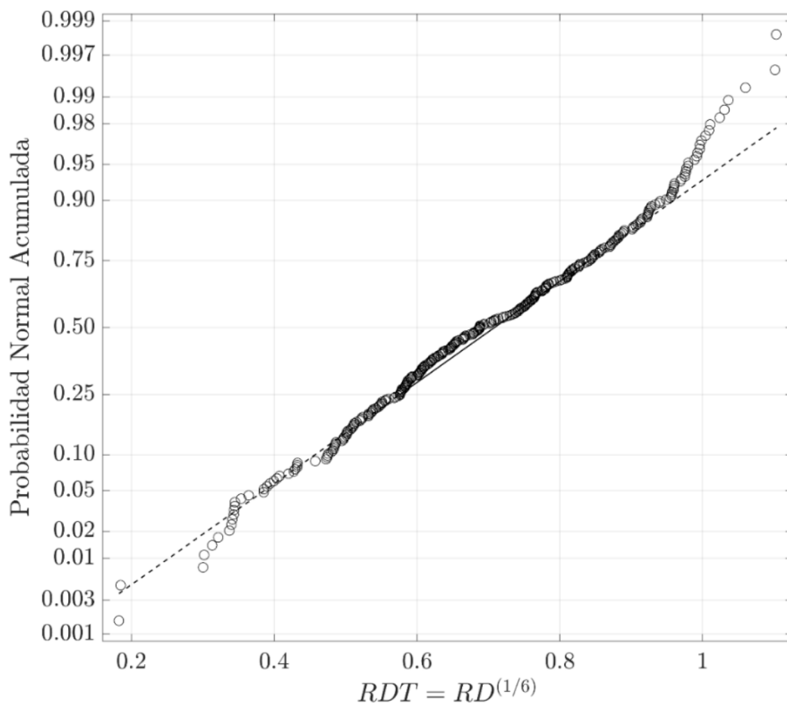
Figura 2 Probabilidad normal acumulada de Fuente: elaboración propia.
