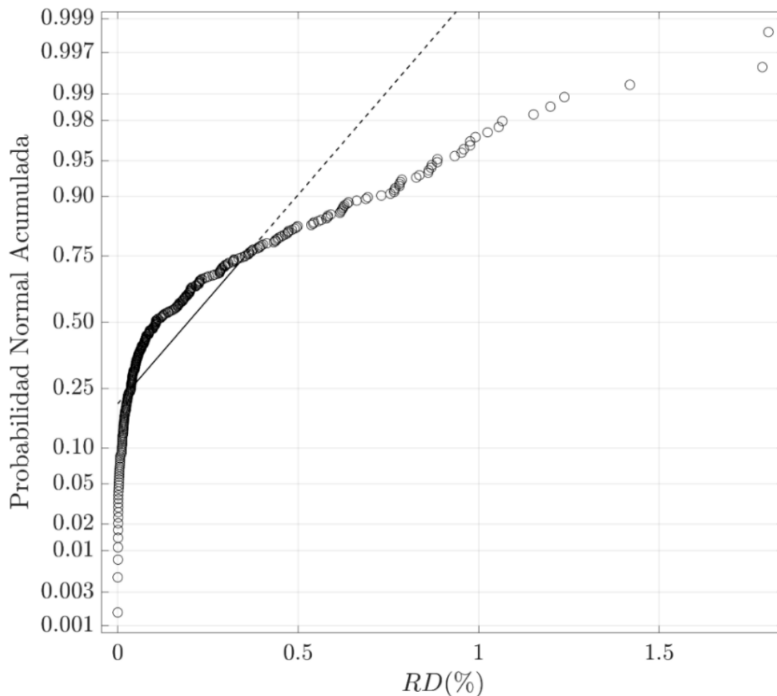
Figura 1 . Probabilidad normal acumulada de Fuente: elaboración propia
