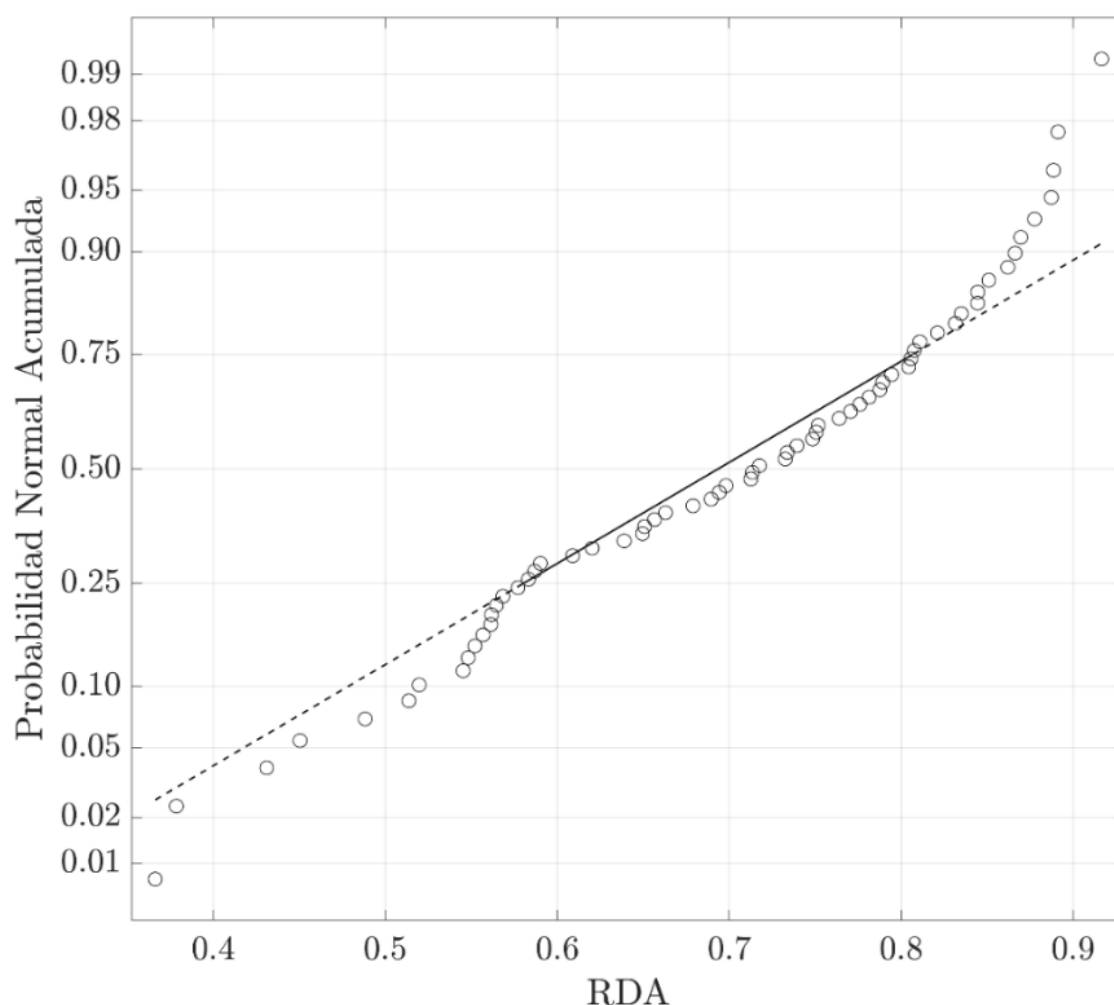
Figura 3 Probabilidad acumulada de RDA. Fuente: elaboración propia.
