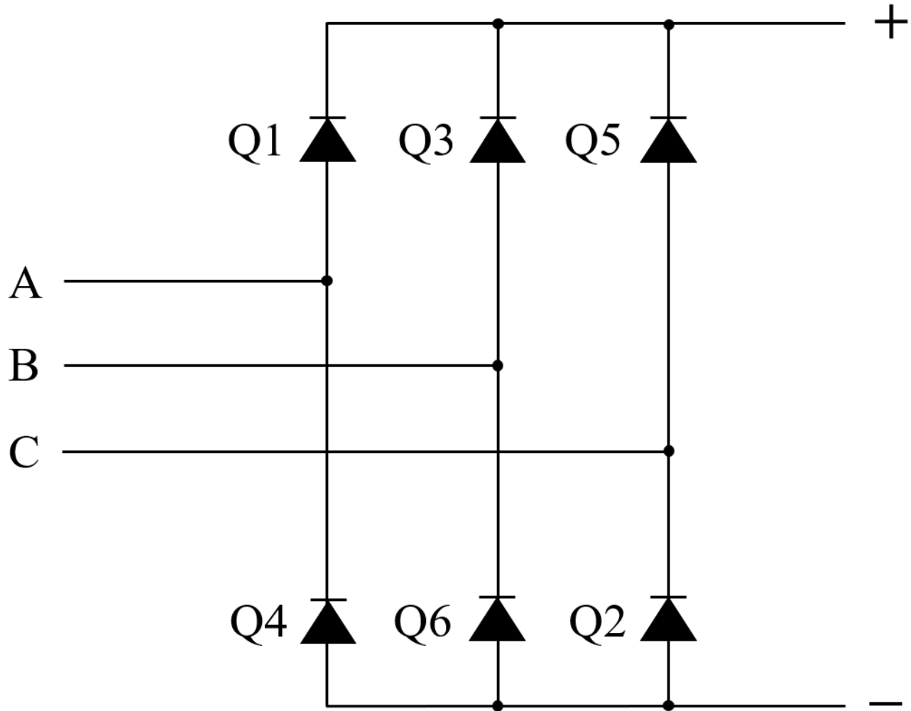
Figura 4. Convertidor AC/DC. Fuente: elaboración propia.
