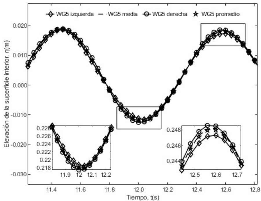
Figura 8. Fluctuaciones de la columna de agua a la derecha, centro e izquierda de la superficie libre bajo el efecto de una ola incidente para las condiciones del océano Pacífico a escala 1:50. Fuente: elaboración propia.
