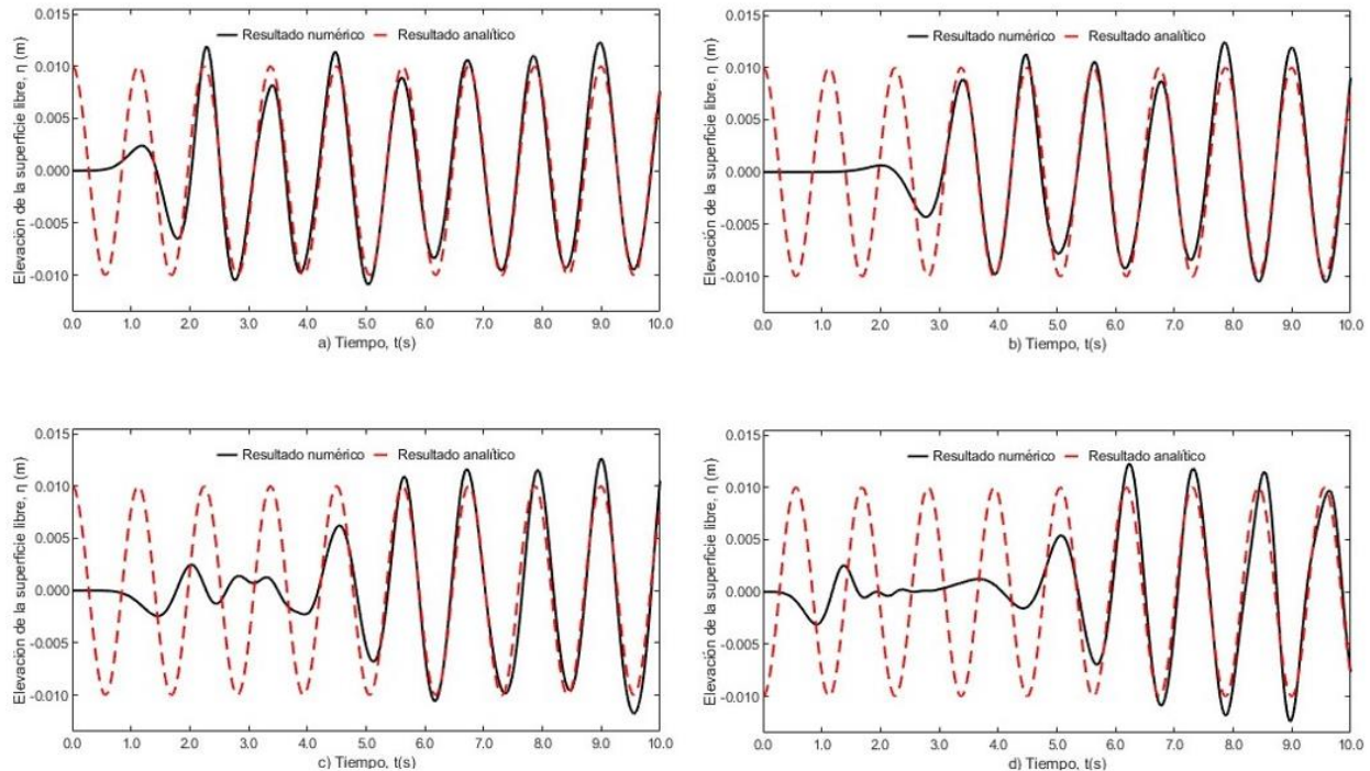
Figura 9. Validación mediante comparación de los resultados numéricos y analíticos obtenidos para una ola de H = 0.02 m a) WG1 a X = \lambda , b) WG2 a X = 1.5\lambda , c) WG3 a X = 2\lambda , d) WG4 a X = 3\lambda
