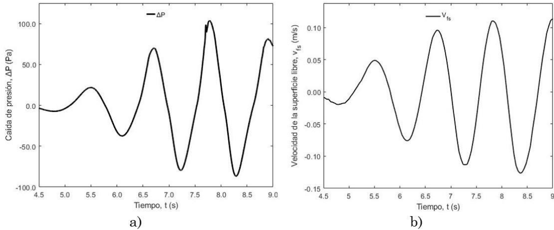
Figura 12. Serie de tiempo de a) presión diferencial, b) velocidad de la columna de agua Fuente: elaboración propia.
