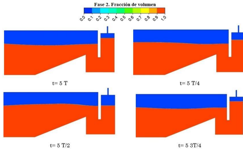
Figura 13. Contorno de fases en instantes de tiempo sucesivos para el tratamiento óptimo. a) el color rojo indica agua, b) el color azul indica aire. Fuente: elaboración propia.
