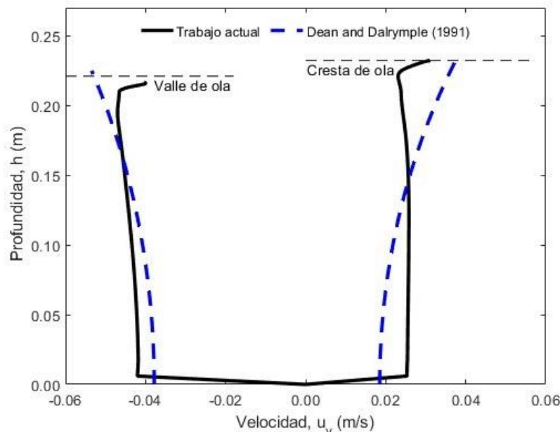
Figura 11. Comparación del perfil de velocidad en la dirección x debajo de la cresta y el valle obtenidos Fuente: elaboración propia.
