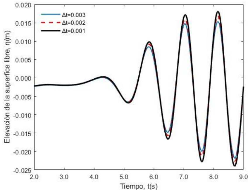
Figura 6. Independencia temporal. Fuente: elaboración propia.
