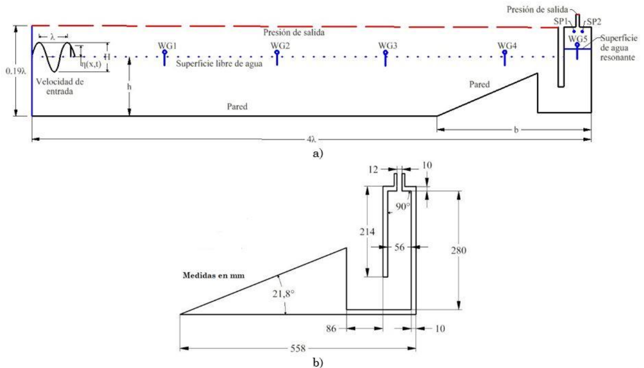
Figura 2. a) Canal de olas para las condiciones del océano Pacífico b) dimensiones de OWC Fuente: elaboración propia.
