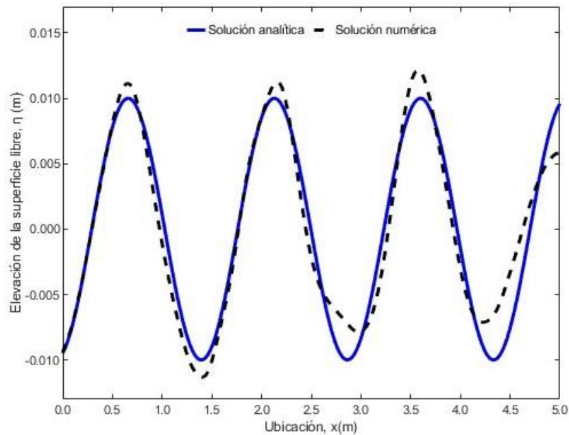
Figura 10. Comparación entre la solución analítica y numérica del frente de ola para las condiciones del Océano Pacífico colombiano. ( H = 0.02 y \lambda = 1.47 metros). Fuente: elaboración propia.
