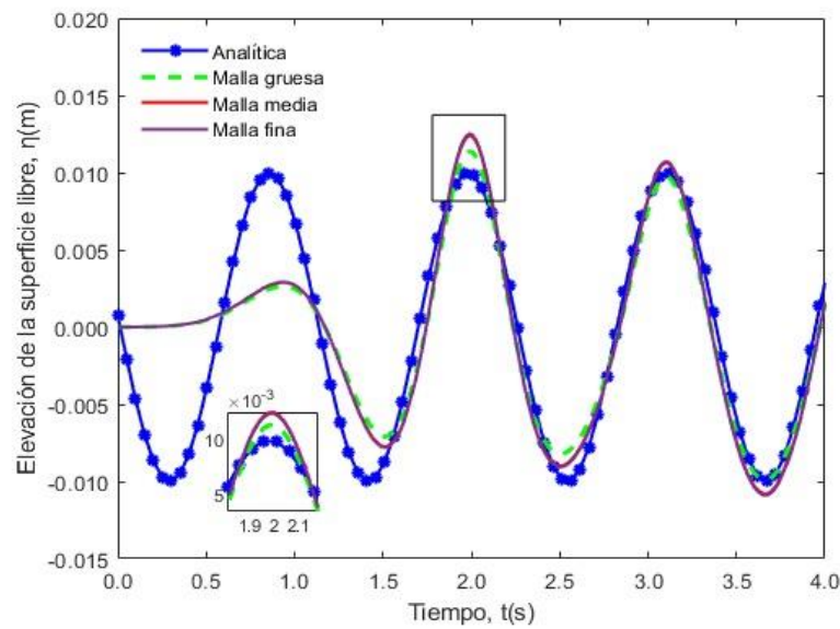
Figura 4. Elevación de la superficie libre a X = \lambda . Fuente: elaboración propia.
