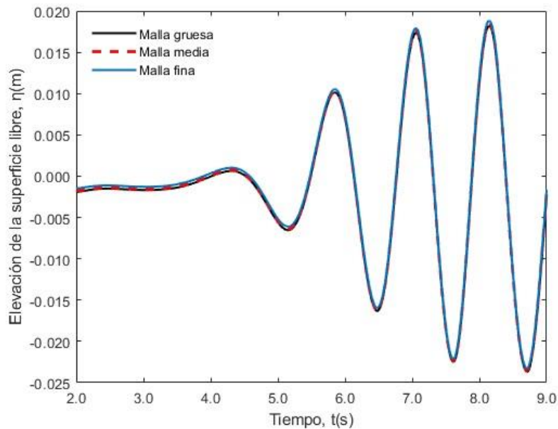
Figura 5. Independencia espacial. Fuente: elaboración propia.
