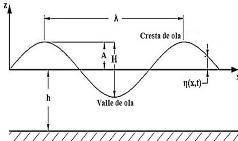
Figura 1. Caracterización de las olas. Fuente: [33].
