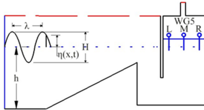
Figura 7. Ubicación de los tres medidores de onda en WG5 (izquierdo, medio y derecho) Fuente: elaboración propia.
