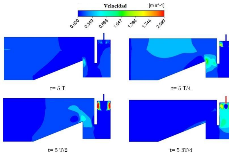
Figura 14. Contorno de líneas de velocidad en instantes de tiempo sucesivos para el tratamiento óptimo Fuente: elaboración propia.
