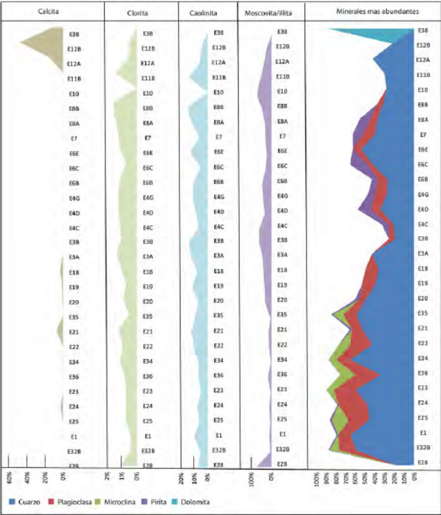
Figura 7. Proporción de los minerales presentes en las muestras (determinados con difracción de rayos X), con los valores normalizados de la altura de los picos para los minerales de arcilla y la calcita.
