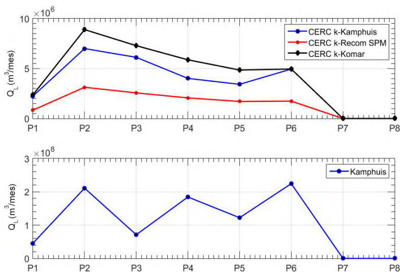
Figura 13. Series de transporte potencial longitudinal de sedimentos a escala medio anual compuesta por las diferentes ecuaciones propuestas.
