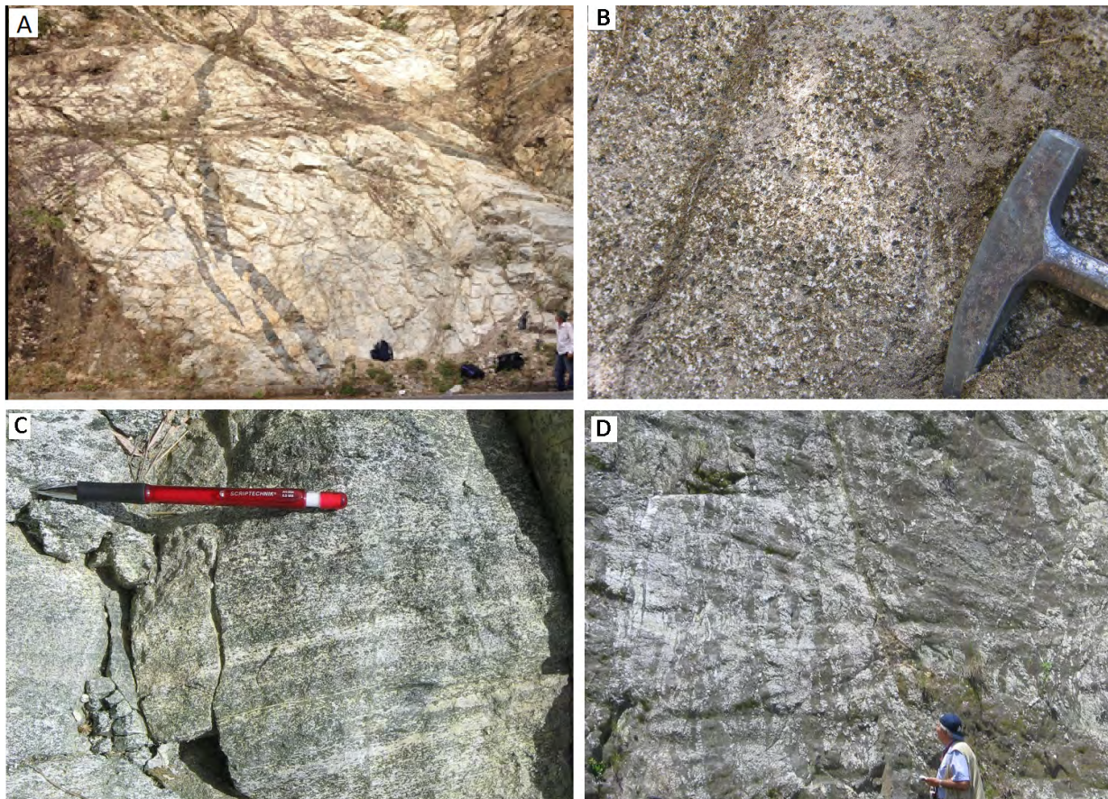
Figura 3. Aspecto macroscópico de algunos plutones. A. Tonalita de Buriticá cortada por diques basálticos. B. Gabro de Caicedo. C. Granulita de Pantanillo con estructura bandeada. D. Tonalita de Santa Fe de Antioquia con xenolitos básicos de gabro hornbléndico rodeados de tonalita y cuarzodiorita.
