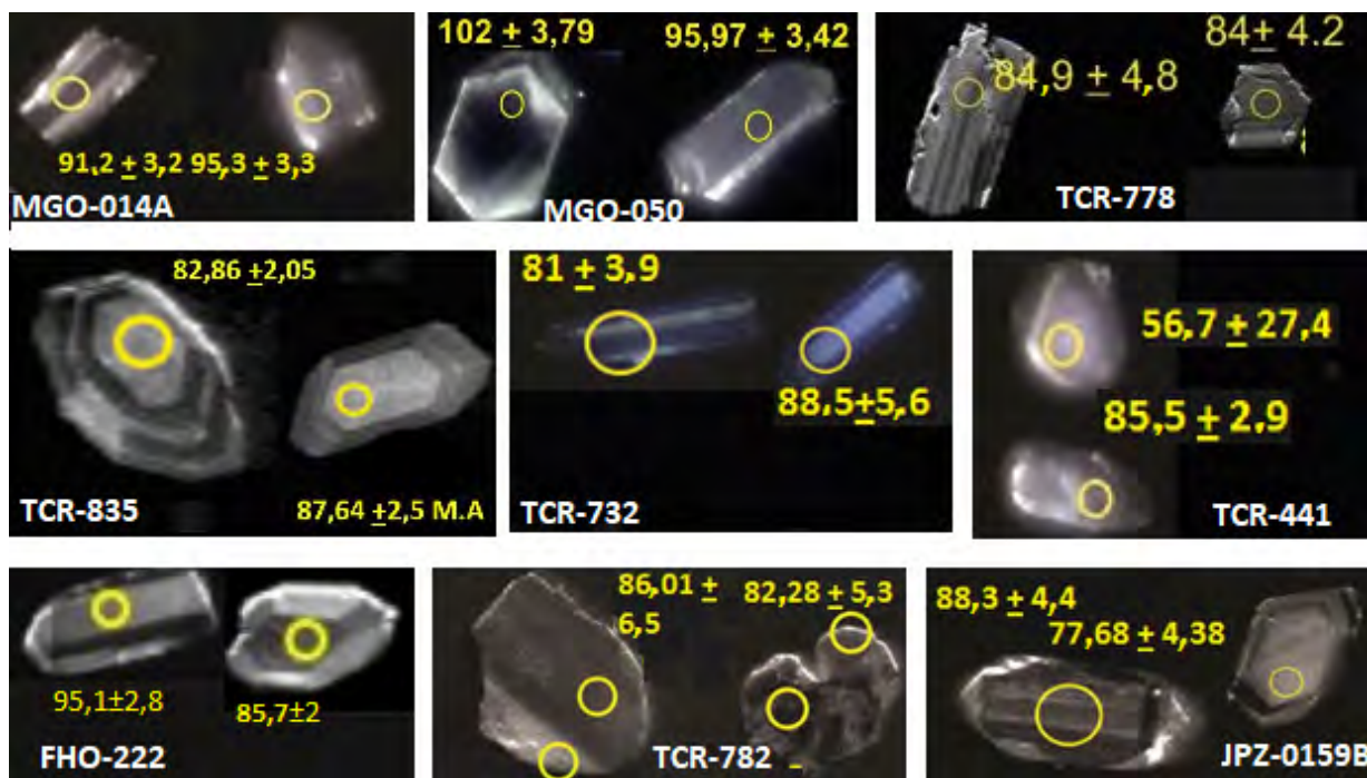
Figura 4. Imágenes de catodoluminiscencia de cristales de circón representativos de muestras datadas de cuerpos del arco insular cretácico. Tonalita de Buriticá (MGO-014A); tonalita de La Noque (MGO-050 y TCR-778), tonalita de Santa Fe de Antioquia (TCR-835, TCR-732 y FHO-222) y granulita de Pantanillo (TCR-441, TCR-782 y JPZ-0159B).
