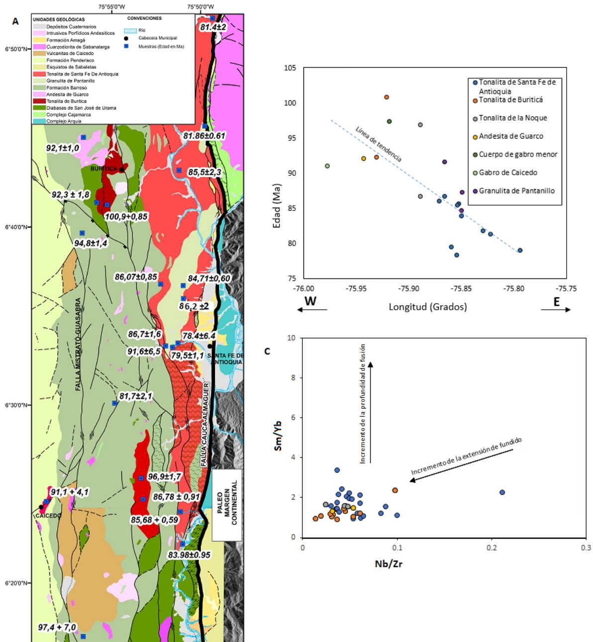
Figura 7. Geología del área de estudio y localización de edades U-Pb en circón en plutones y vulcanitas del ABS, junto con un diagrama de edad vs longitud y Nb/Zr vs Sm/Yb (He et al. , 2010).
