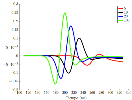
Figura 5. Formas de las ondulitas a una distancia de (4000 m, 4000 m) de la fuente, para los medios con diferentes valores de Q .
