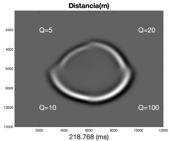
Figura 4. Instantánea de las ondulitas en un medio homogéneo de velocidad con diferentes valores de Q .
