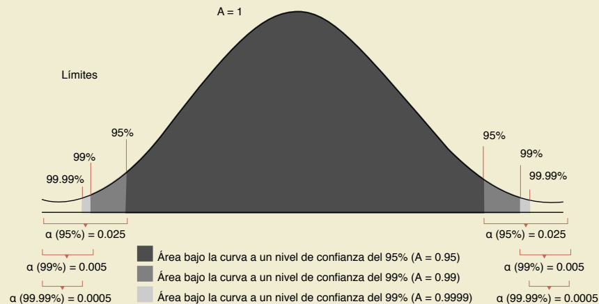
Figura 2. Ilustración de la función matemática de Gauss de una variable con distribución normal, los límites de intervalos de confianza al 95%, 99% y 99.99%, así como los valores \alpha correspondientes a cada nivel de confianza
