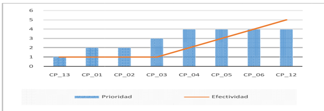
Fig. 5. Resultados para las pruebas de la caja negra escenario 1
