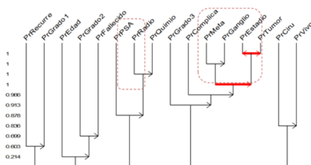
Fig. 2. Relaciones causales entre factores pronósticos (árbol cohesitivo)
