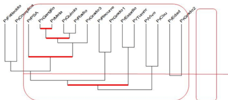
Fig. 1. Árbol de similaridad
