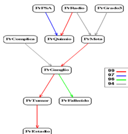
Fig. 3. Grafo implicativo de las relaciones causales entre los factores pronóstico con 95 % y más de intensidad implicativa.
