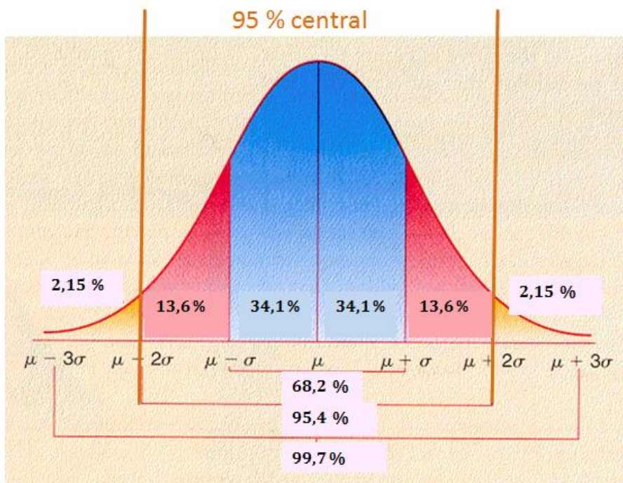
Fig.2. Curva de Gauss
