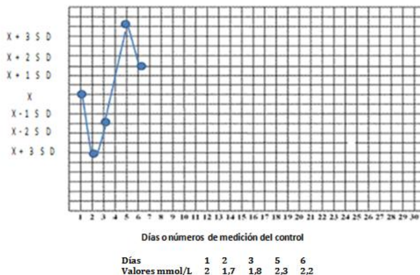
Fig. 1. Ejemplo del uso de la gráfica de Levey Jennings con 5 valores de suero control de colesterol, obtenido en condiciones óptimas \bar{X}=2 mmol/L SD=0,1 mmol/L
