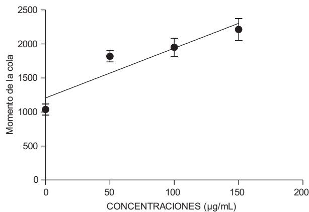
Fig. 2. Relación concentración unidades arbitrarias de daño al ADN tras exposición a distintas concentraciones (µg/mL) de la formulación comercial de glifosato II (Atanor®). Coeficiente de correlación r = 0.9342 , p = 0.0329 , prueba de Pearson.
