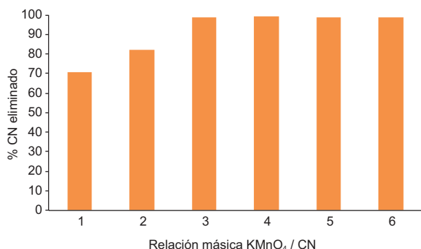
Fig. 3. Eliminación de cianuro (CN) del agua residual CIL (concentración inicial de cianuro de 312 mg/L) en función de la relación másica \text{KMnO}_4 /CN.
