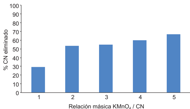
Fig. 5. Eliminación de cianuro (CN) del agua de drenaje (concentración inicial de cianuro de 1.9 mg/L) en función de la relación másica \text{KMnO}_4 /CN.
