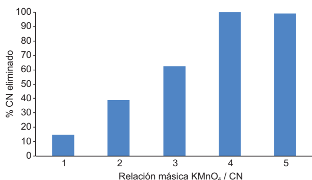
Fig. 4. Eliminación de cianuro (CN) de agua de proceso pre-tratada con \text{SO}_2 (concentración inicial de cianuro de 15 mg/L) en función de la relación másica \text{KMnO}_4 /CN.
