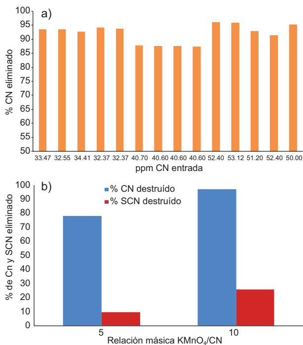
Fig. 6. (a) Eliminación de cianuro en agua de proceso recogida en continuo para una relación másica \text{KMnO}_4 /CN de 5:1; pH = 12 y 20 min de agitación. (b) Eliminación de cianuro y tiocianato en el agua de proceso recogida en continuo para relaciones másicas \text{KMnO}_4 /CN de 5 y 10, pH= 12 y 20 min. de agitación.
