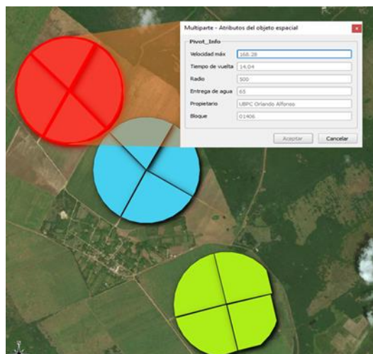
Figura 5. Mapa temático de características técnicas de máquina de riego de pivote central Cuñat Agrocaja
