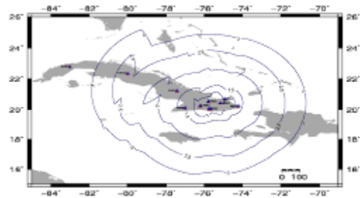
Figura 10. Umbral de detección real efectivo suavizado usando el algoritmo propuesto para las 11 estaciones, año 1999.
