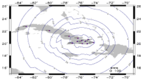
Figura 13. Umbral de detección para el territorio de Cuba con las 12 estaciones existentes en el año 2014.
