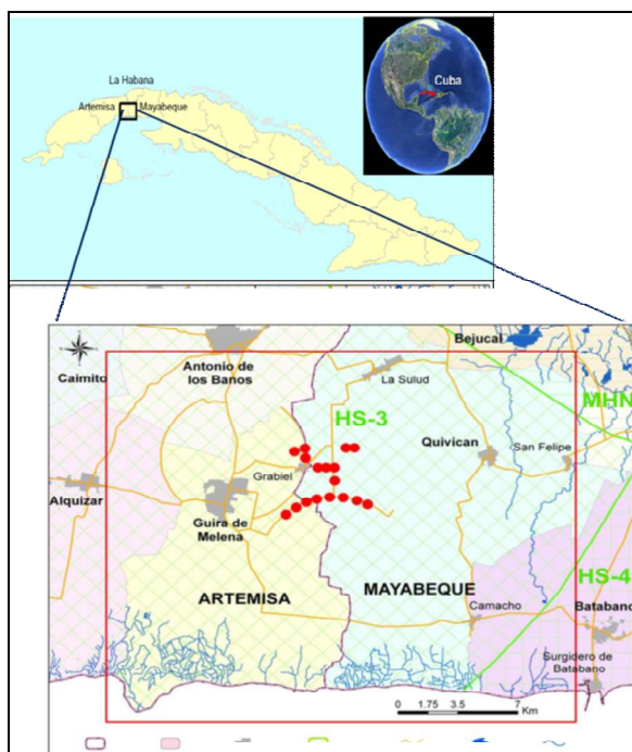
Figura 1. Ubicación del área de estudio en la Cuenca Sur de Artemisa y Mayabeque.
