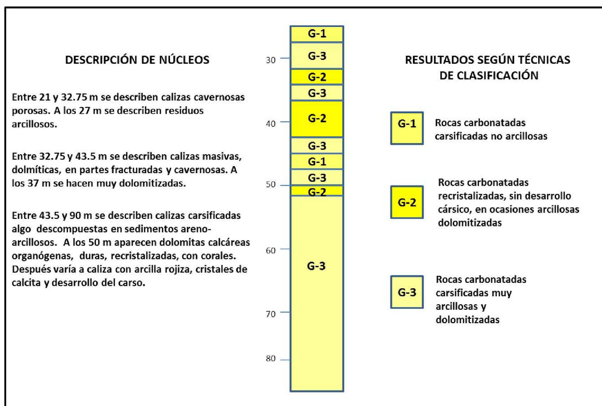
Figura 3. Clasificación litológica propuesta como resultado de aplicar el Análisis Euclidiano de Agrupación y descripciones de núcleos disponibles en la sala I-II-12K de la Cuenca Sur de las provincias Artemisa y Mayabeque.
